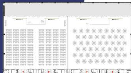
CH3,4 1/2 スクール 2名掛480席
